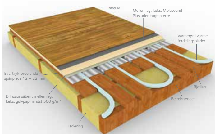
Eksempel på opbygning med bærebærdæder og varmfordelingsplader.
